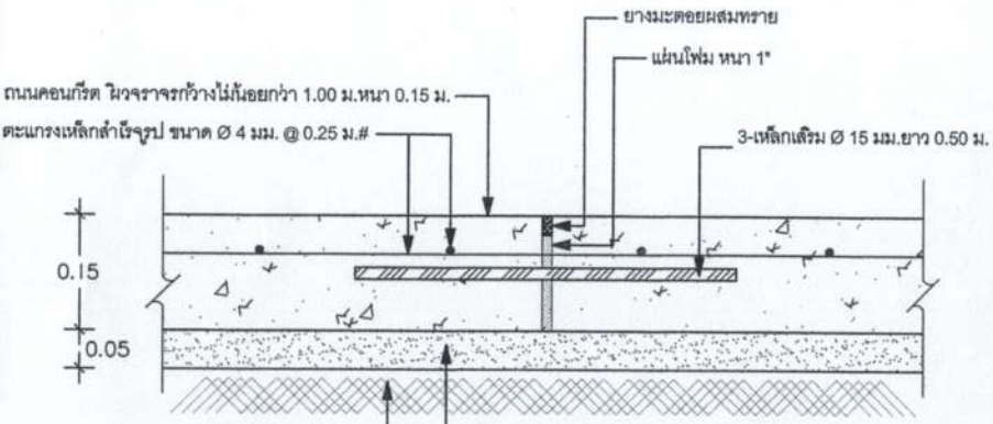
รูปตัดถนน (C)
